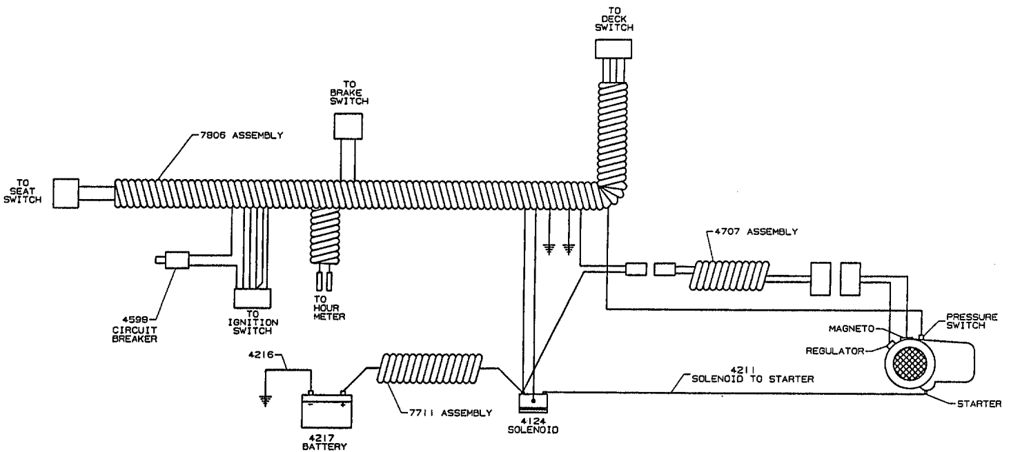
BODY WIRING LOOM 7806 WIRING KIT 8809
